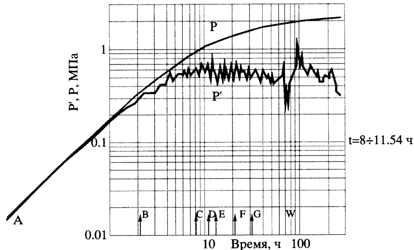
Рисунок А9. Диагностический бипологарифмический график ГДИС горизонтальной скв. 11412 КВД-1. Буквы – диагностические участки.
