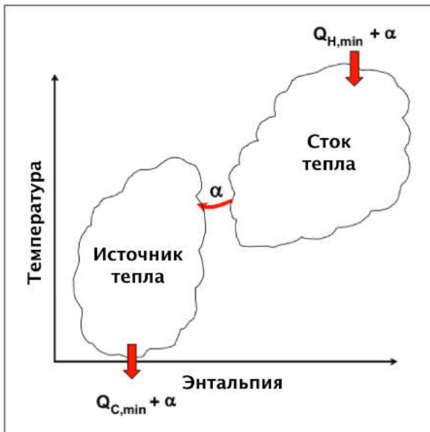
Рисунок 2.15: Передача тепла через пинч от стока к источнику
