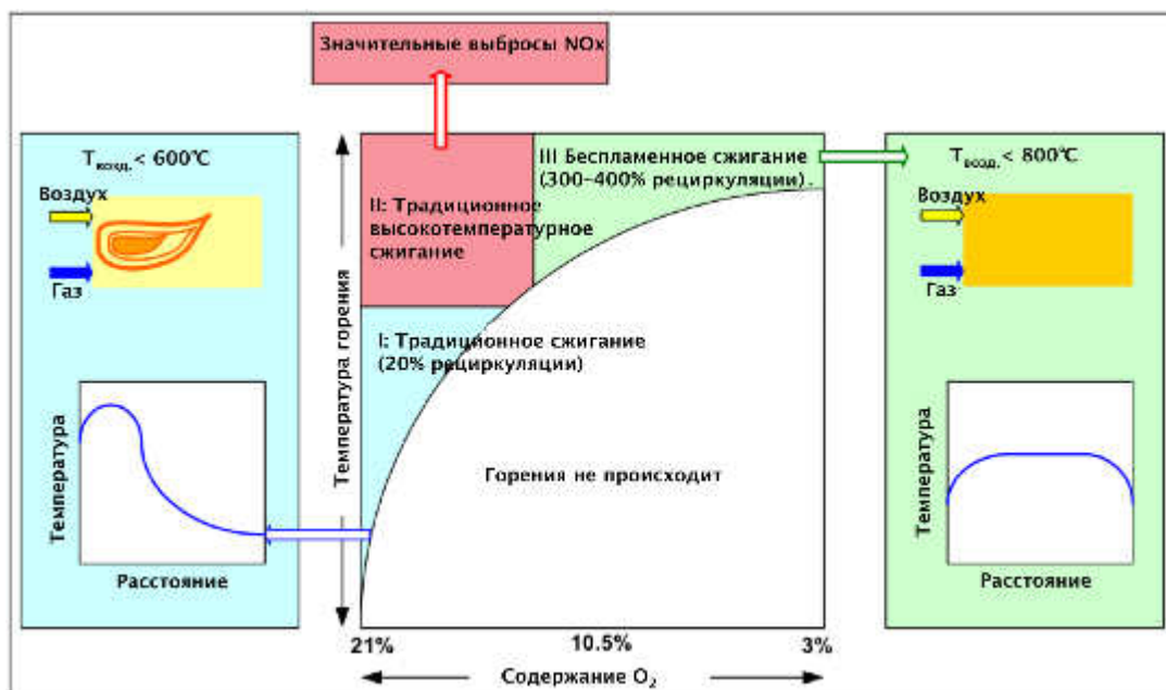
Рисунок 5.3: Условия беспламенного сжигания
