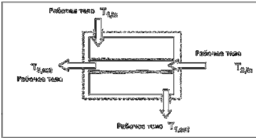
Рисунок 7.4: Противоточный теплообменник
