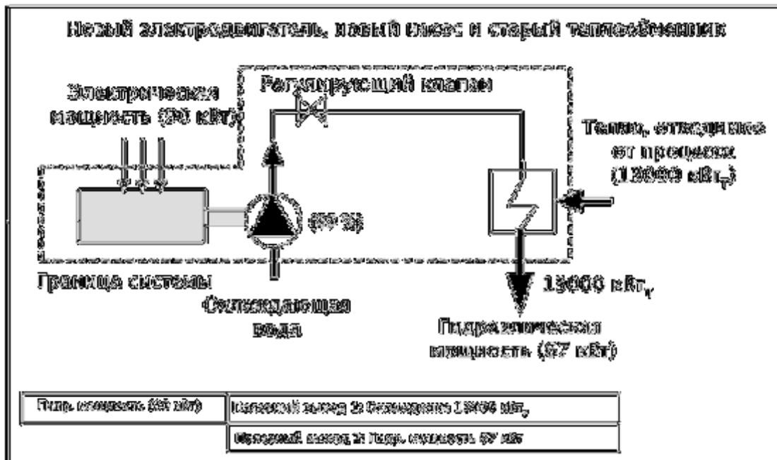
Рисунок 1.15: Новый электродвигатель, новый насос и старый теплообменник
