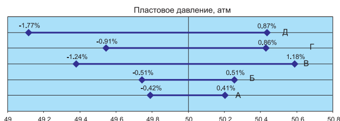
Рис. 6. Интервальная оценка пластового давления по вариантам А, Б, В, Г, Д при максимальной невязке \Delta P=0.05 атм. Фактическое значение – 50 атм.
