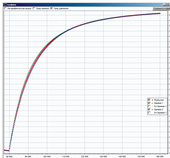
Рис. 2. Результаты интерпретации по варианту Г (не учитывается переходной участок).
