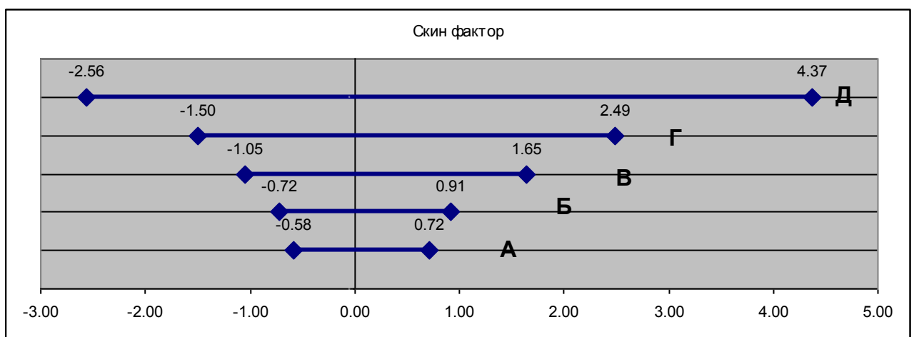
Рис. 9. Интервальная оценка скин-фактора по вариантам А, Б, В, Г, Д при максимальной невязке \Delta P=0.05 атм. Фактическое значение – 0.
