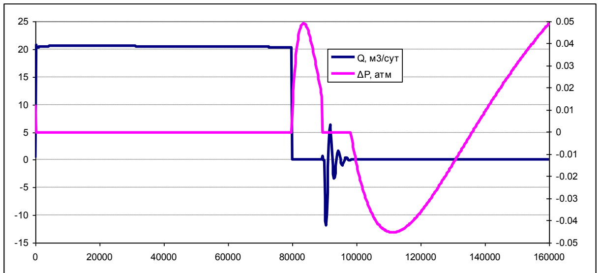
Рис. 5. Результаты интерпретации по варианту Б (со скачками давления). Показаны: погрешность аппроксимации, не превышающая 0.05 атм, и модельное значение дебита, рассчитанное на участках, интерпретированных в режиме заданного давления. Погрешность аппроксимации давления на этих участках равна 0.
