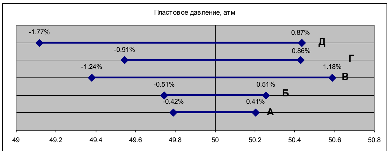
Рис. 6. Интервальная оценка пластового давления по вариантам А, Б, В, Г, Д при максимальной невязке \Delta P=0.05 атм. Фактическое значение – 50 атм.
