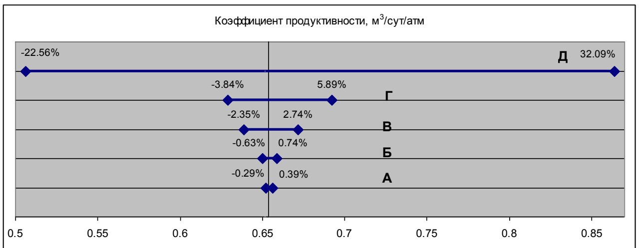
Рис. 8. Интервальная оценка коэффициента продуктивности по вариантам А, Б, В, Г, Д при максимальной невязке \Delta P=0.05 атм. Фактическое значение – 0.6539 м³/сут/атм.
