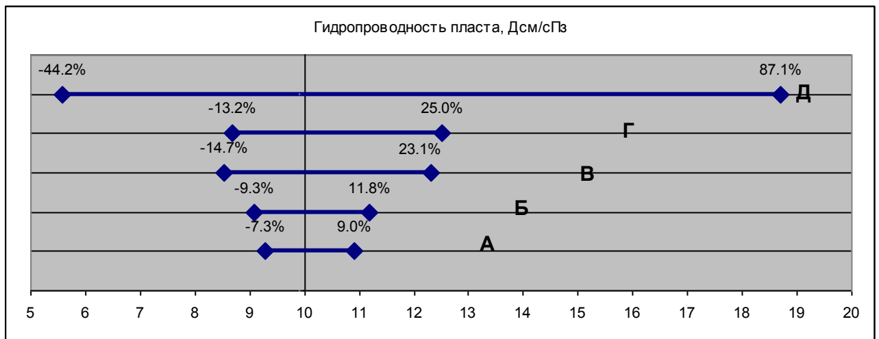
Рис. 7. Интервальная оценка гидропроводности пласта по вариантам А, Б, В, Г, Д при максимальной невязке \Delta P=0.05 атм. Фактическое значение – 10 Д*см/спз.
