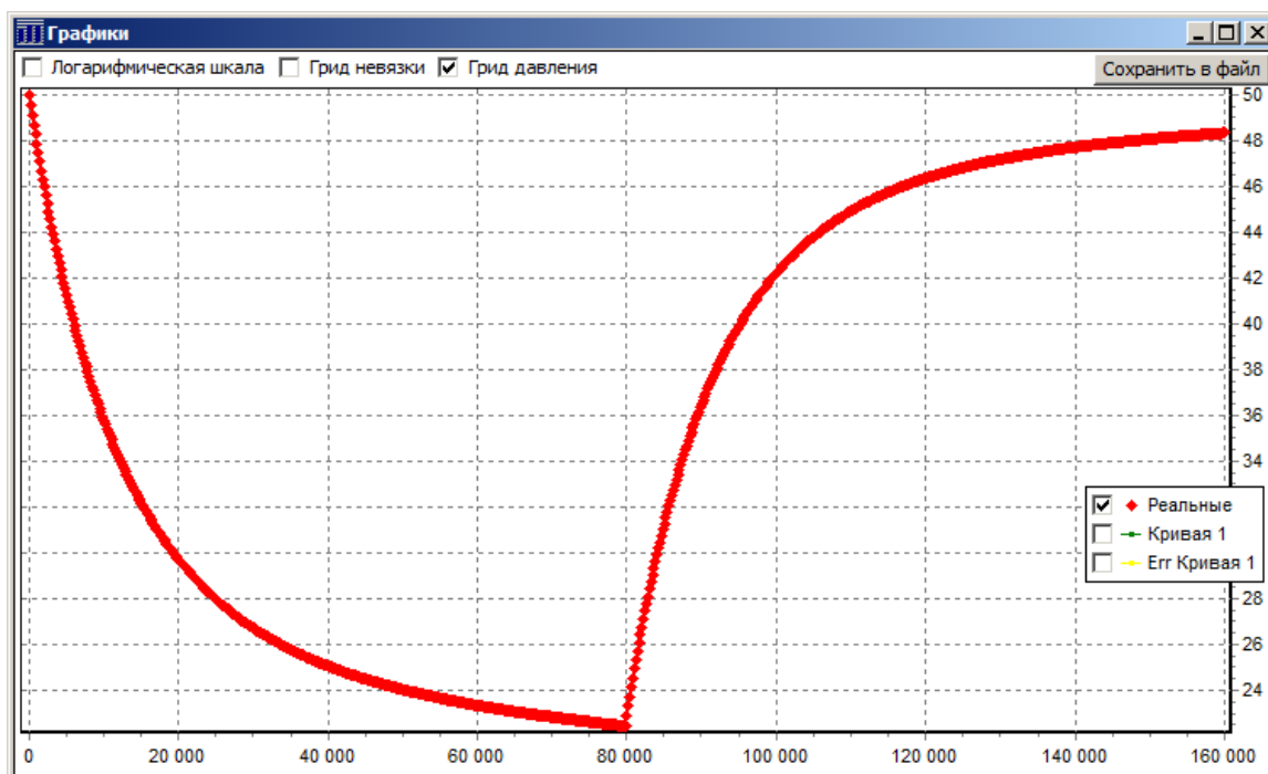
Рис. 1. "Фактическая" кривая изменения давления модельной системы: от 0 до 80000 сек скважина работает с дебитом 20 м 3 /сут.; от 80000 до 160000 сек скважина остановлена.
