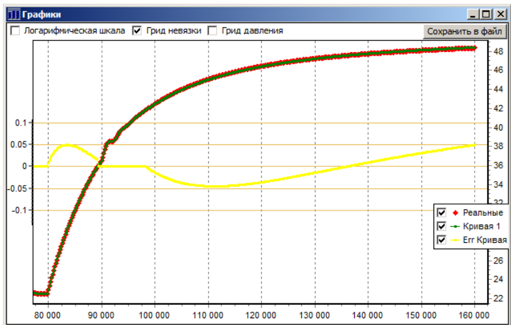
Рис. 4. Результаты интерпретации по варианту Б.
